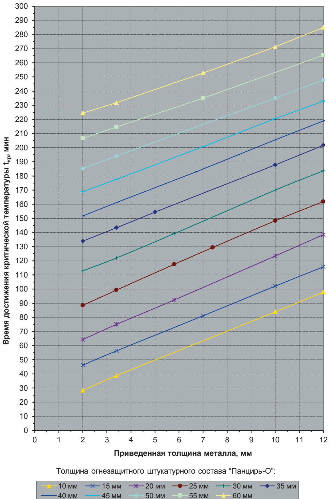
Рис. 19. Огнестойкость стальных конструкций с огнезащитным штукатурным составом "Панцирь-О" при t_{кр} = 450 °С.
