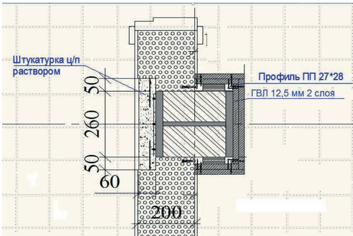
Рис. А23. Принципиальная схема облицовки стальной колонны, находящейся в составе ограждающей конструкции, листовыми материалами типа ГКЛ (ГВЛ, ГКЛО) в два слоя (ограждающая стеновая конструкция показана условно)
