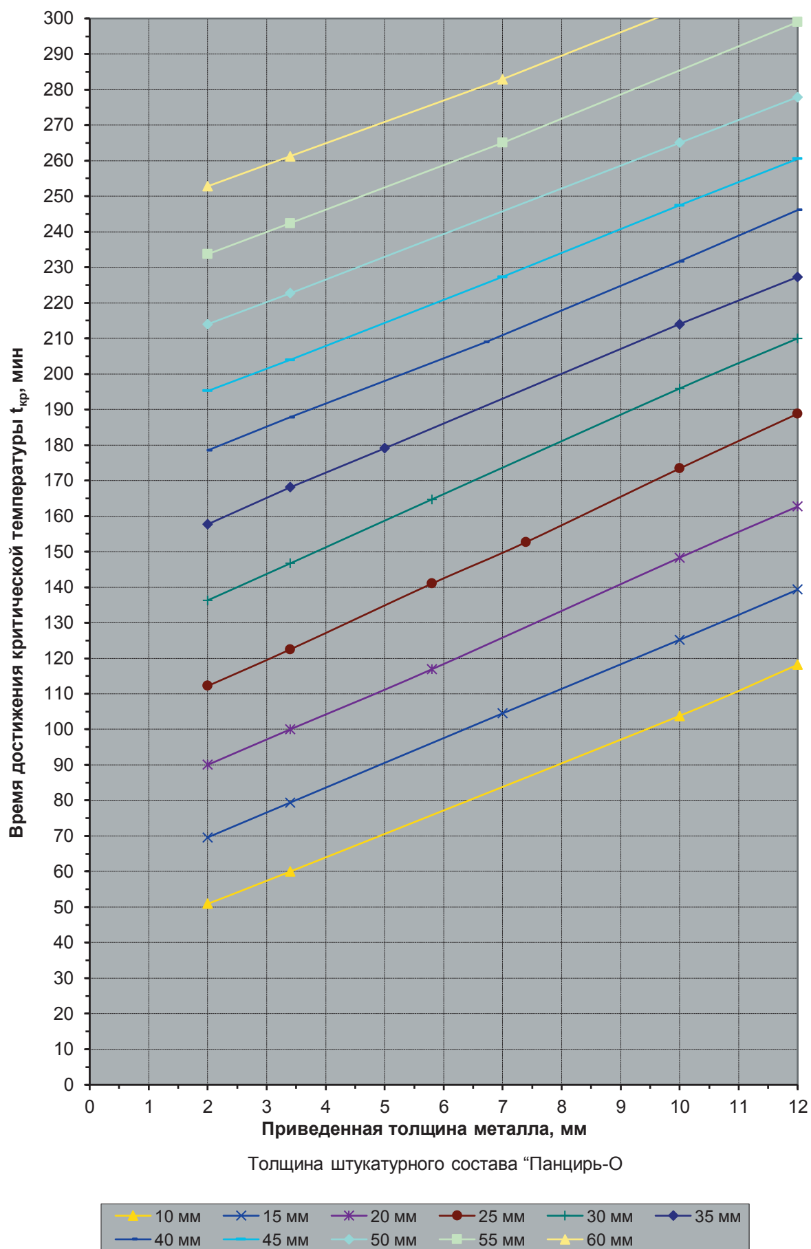
Рис. 22. Огнестойкость стальных конструкций с огнезащитным штукатурным составом «Панцирь О» при t_{кр} = 600^\circ\text{C} .
