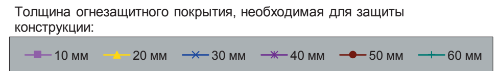
Рис. 18. Огнестойкость стальных конструкций с огнезащитной облицовкой из цементно-песчаной штукатурки при t_{кр} = 600 \text{ }^{\circ}\text{C} .
