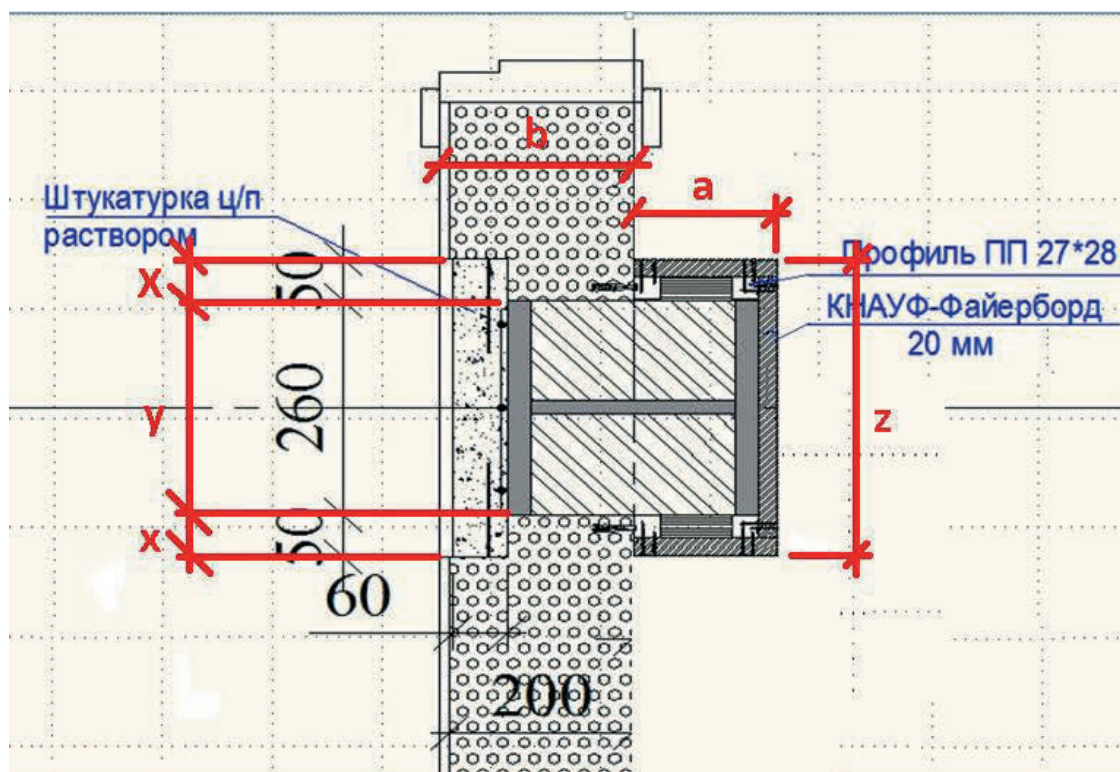
Рис. А24. Принципиальная схема облицовки стальной колонны, находящейся в составе ограждающей конструкции, листовыми материалами типа ГКЛ (ГВЛ, ГКЛО) в один слой (ограждающая стеновая конструкция показана условно)
