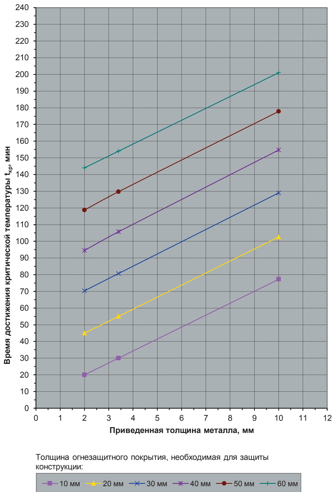
Рис. 15. Огнестойкость стальных конструкций с огнезащитной облицовкой из цементно-песчаной штукатурки при t_{кр} = 450 \text{ }^{\circ}\text{C} .
